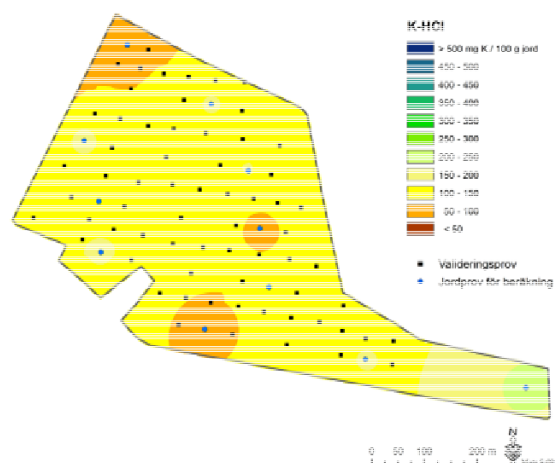
d) Ett prov / 3 ha; IDW exp 1; RPD = 1,11
