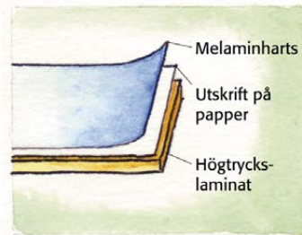
Perstorpsskyltens uppbyggnad.
